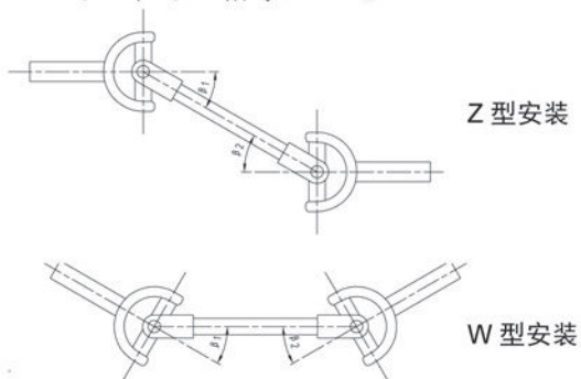
图 1 可实现同步运转的万向轴安装方式
