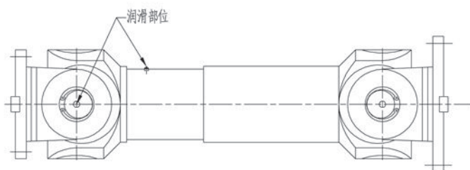
图 2 万向轴的润滑部位
