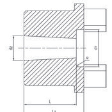
Z 1 型无沉孔的短圆锥型轴孔
