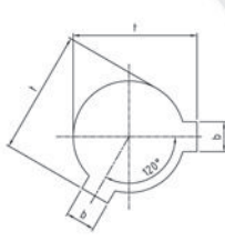
B 型 120 度布置平键双键槽
