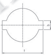
B 1 型 180 度布置平键双键槽
