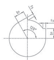
D 圆柱型孔普通切向键键槽
